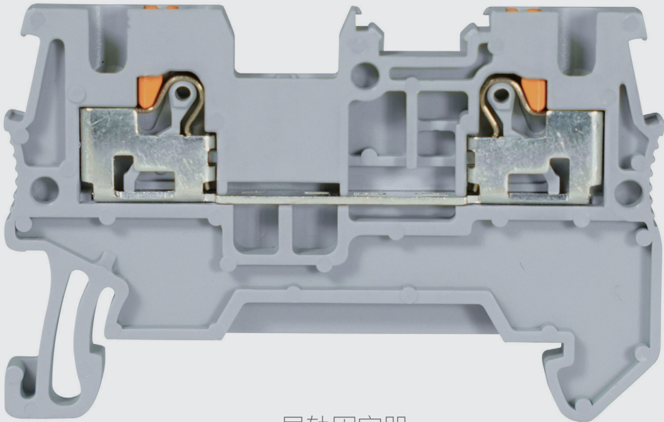
导轨固定器 End clampp
